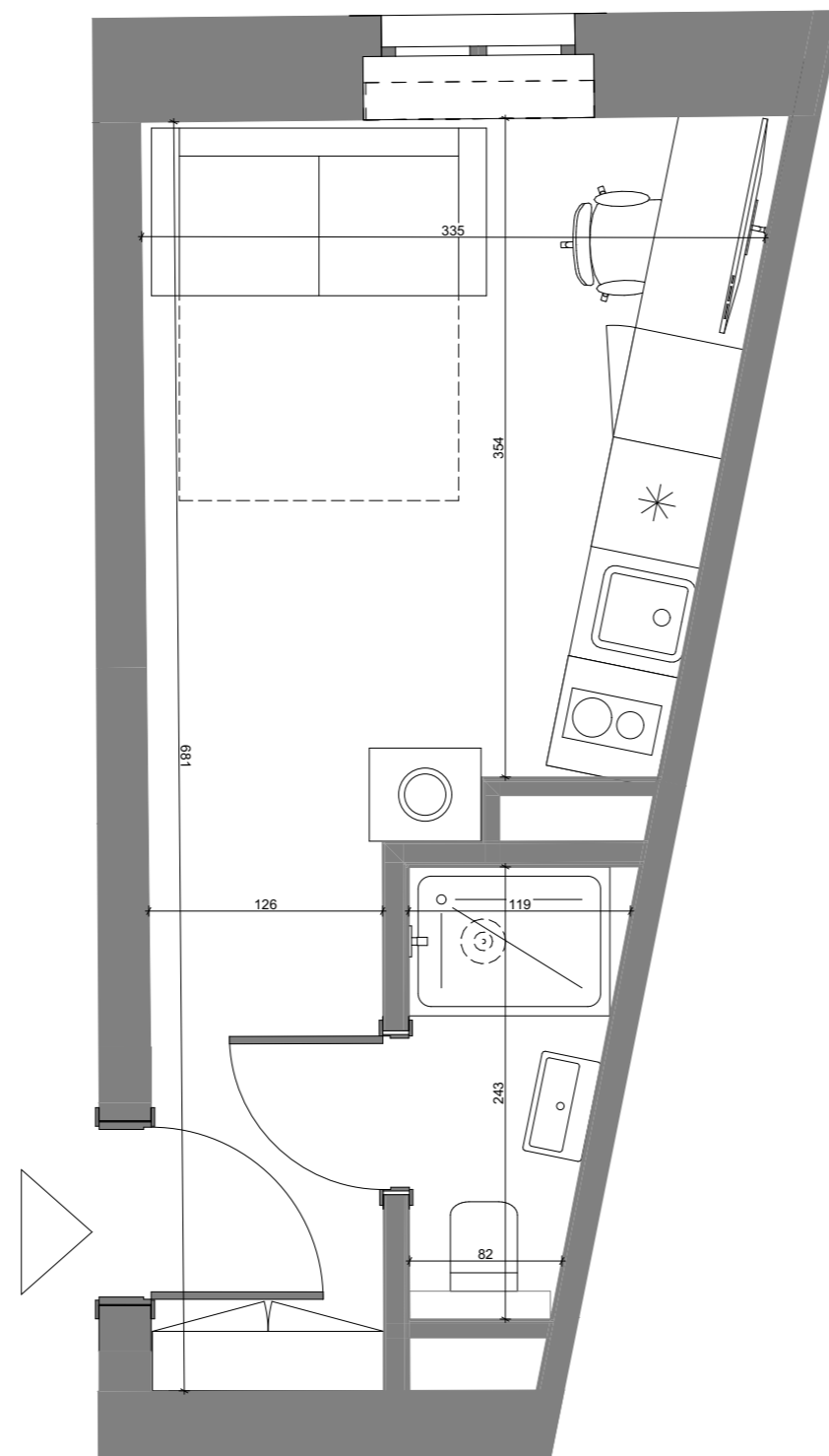
PLAN SYTUACYJNY, SKALA 1:40
