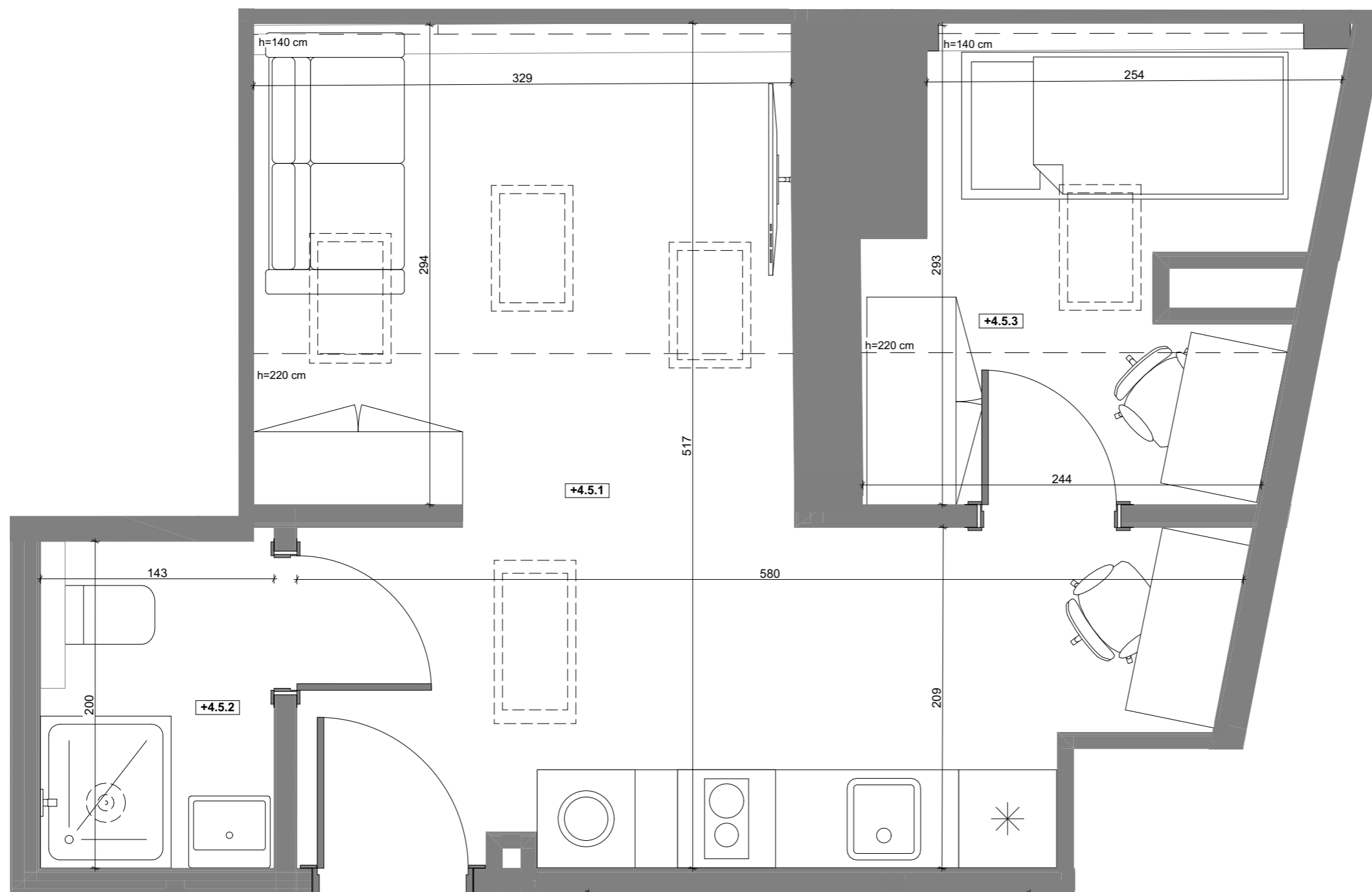
PLAN SYTUACYJNY, SKALA 1:30
